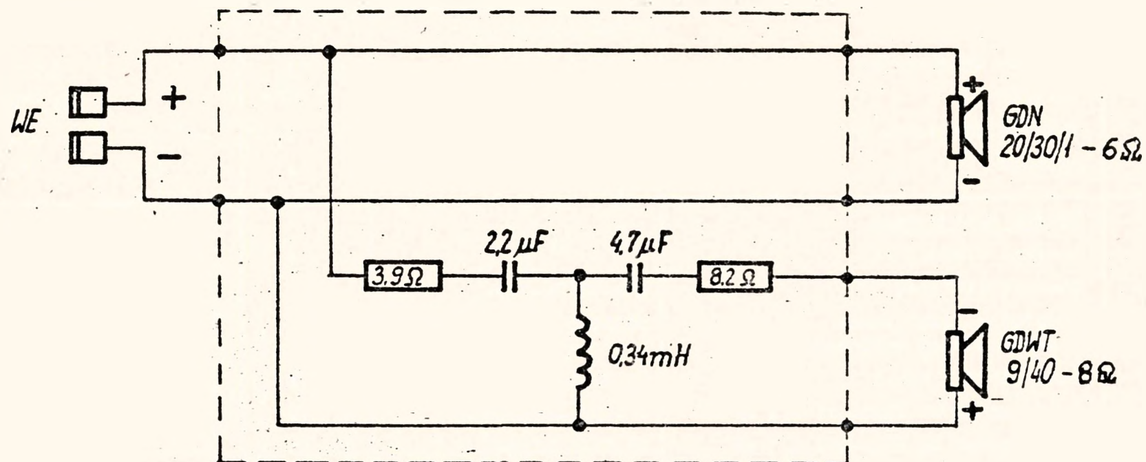
Rys.6 Schemat elektryczno-montażowy zestawu głośnikowego ZG 386
