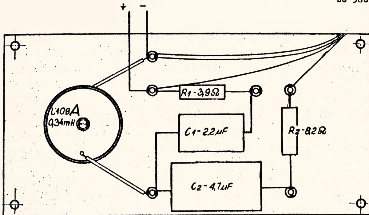
Rys.3 Zwrotnica elektryczna ZQ 386
