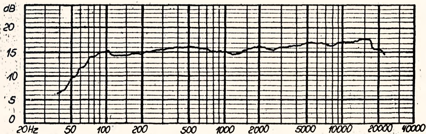
Rys. 1 Przykładowa charakterystyka ośnienia akustycznego zestawu głośnikowego
