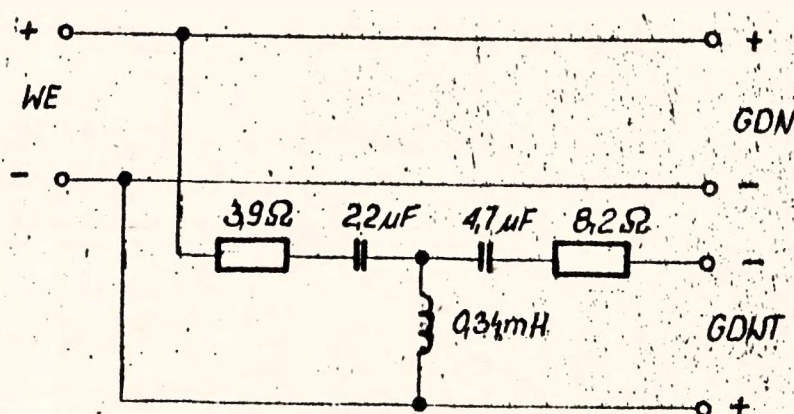
Rys.4 Schemat elektryczny zwrotnicy ZQ 386
