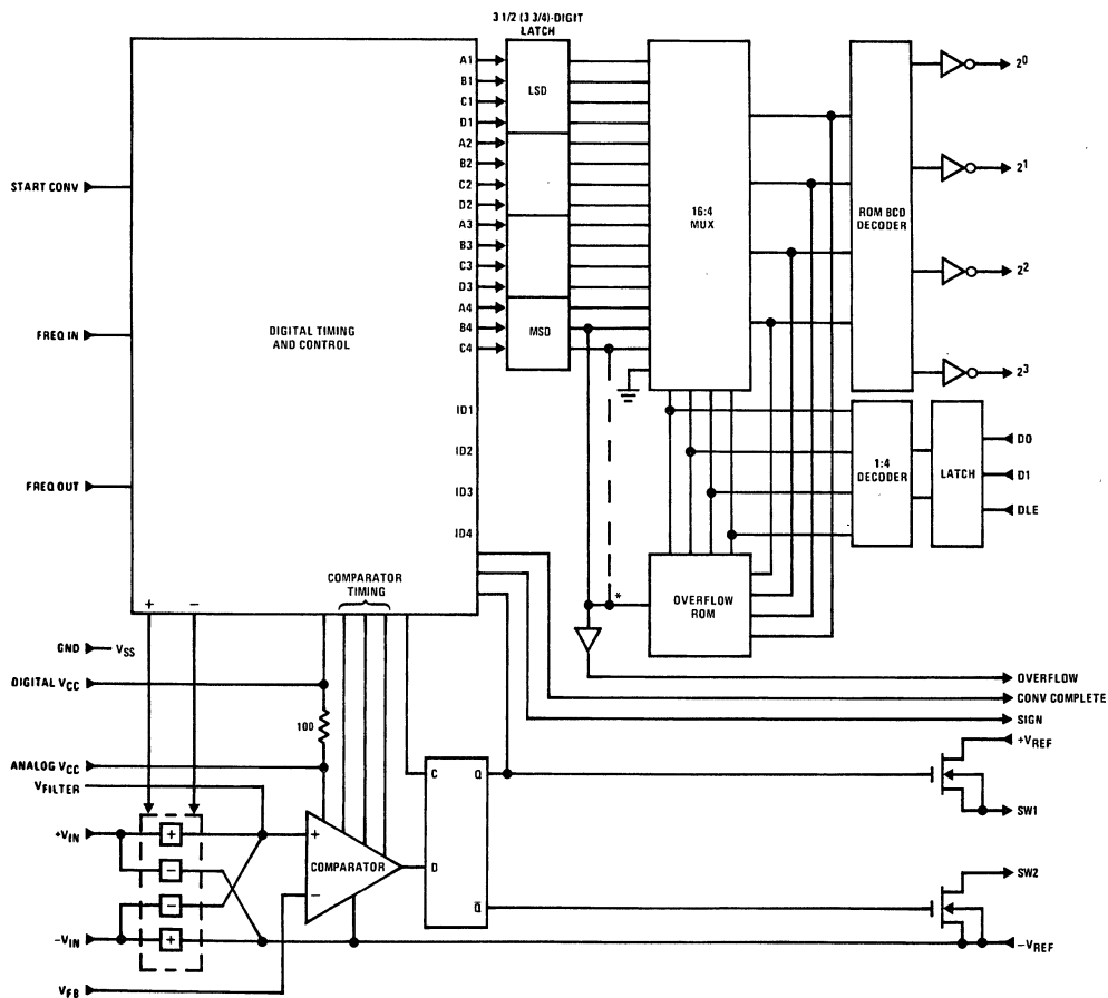
ADC3511 3 \frac{1}{2} -Digit A/D (*ADC3711 3 \frac{3}{4} -Digit A/D)
