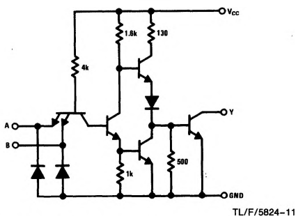
DS55451/DS75451
