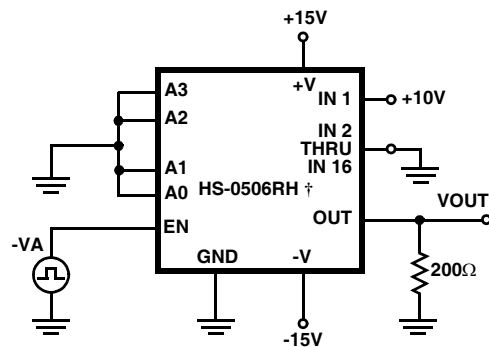
FIGURE 3. ENABLE DELAY t_{ON(EN)} , t_{OFF(EN)}
