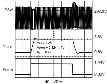
V CON Voltage Response
