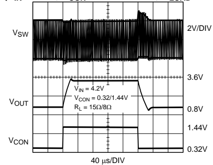
V CON and Load Transient
