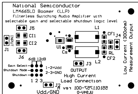
Figure 19. Top Layer
