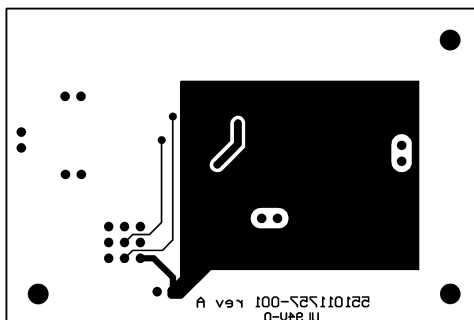
Figure 20. Bottom Layer
