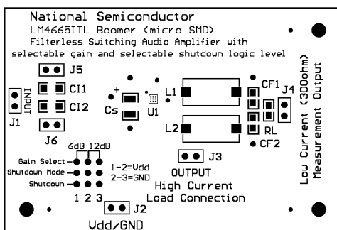
Figure 23. Top Layer
