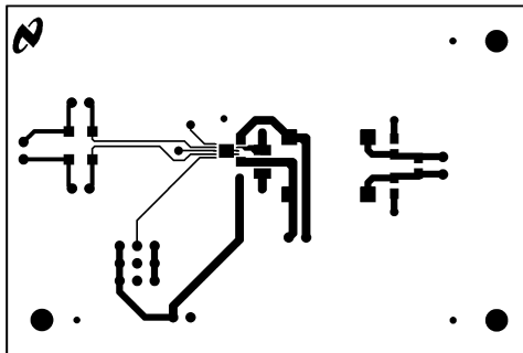
Figure 19. Top Layer
