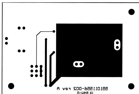
Figure 24. Bottom Layer
