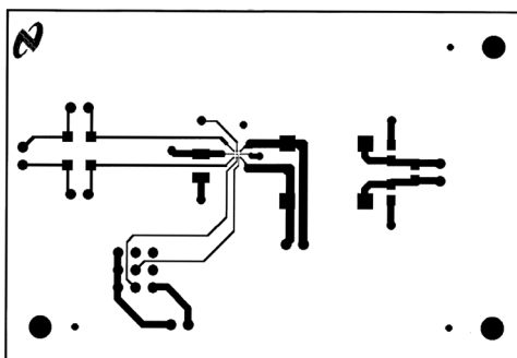
Figure 23. Top Layer
