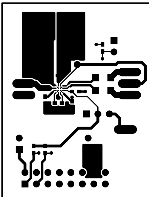
Figure 16. Top Layer
