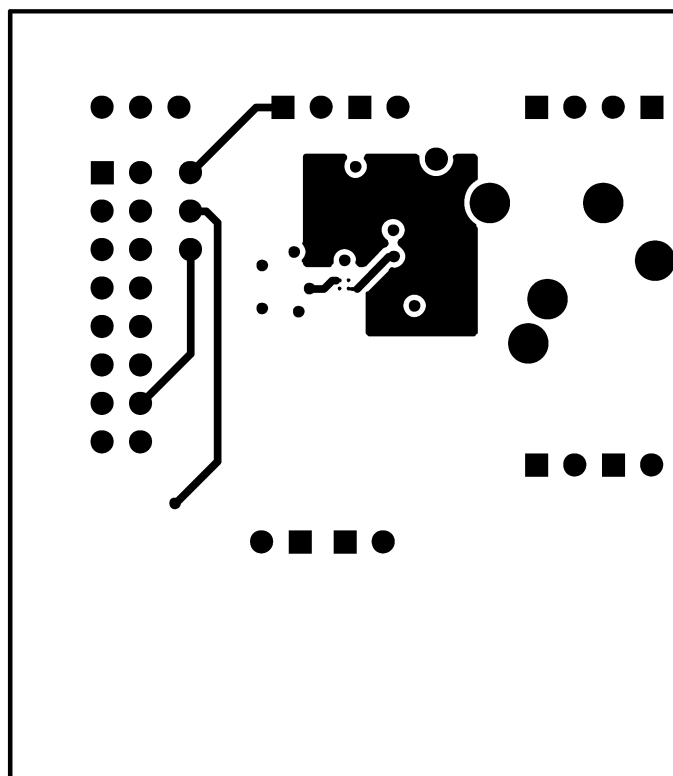
Figure 16. Layer 3 (VDD)
