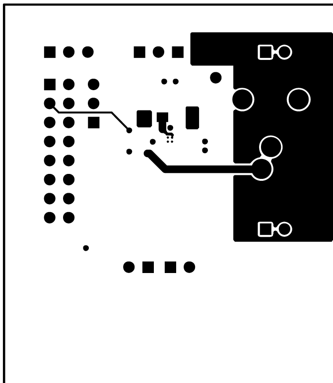
Figure 17. Bottom Layer
