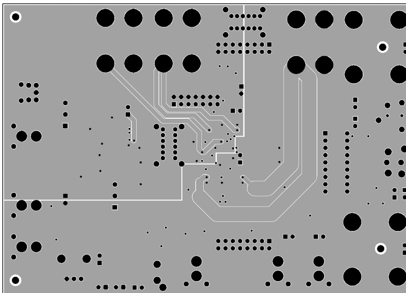
Figure 27. Bottom Layer
