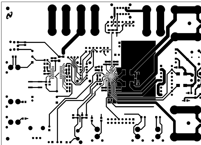
Figure 24. Top Layer
