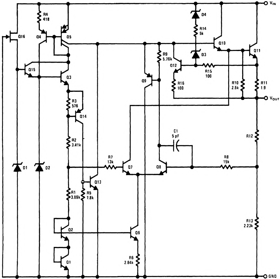
LM78LXX
