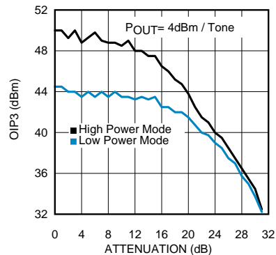
OIP3 vs Attenuation
