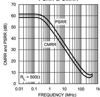
PSRR & CMRR
