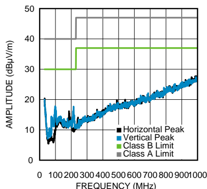
Figure 4. Radiated EMI (EN 55022)
