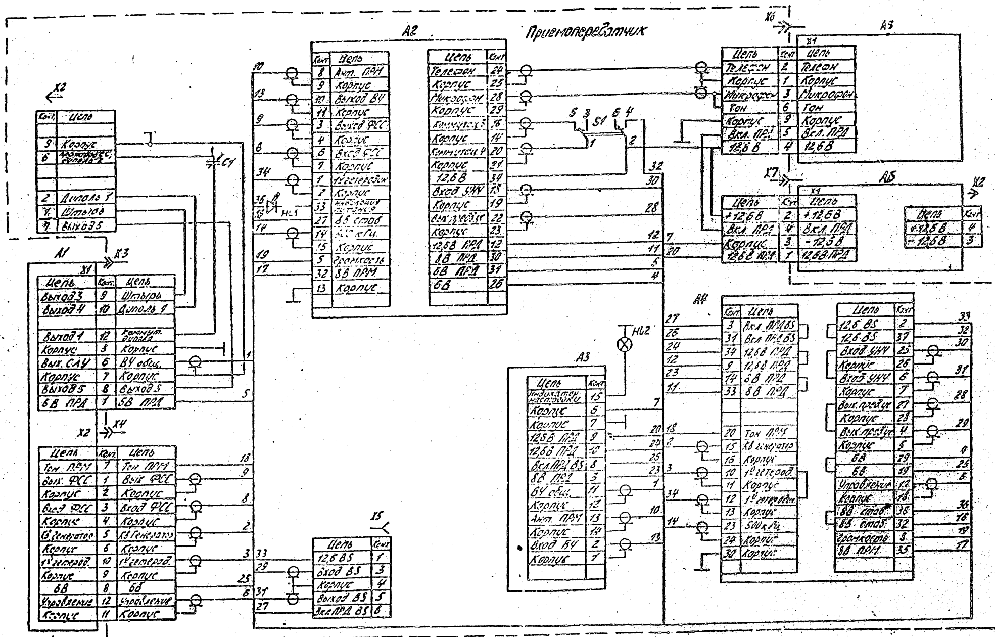
ИЗДЕЛИЕ „СЕВЕРОК-К“. СХЕМА ЭЛЕКТРИЧЕСКАЯ ПРИНЦИПИАЛЬНАЯ
