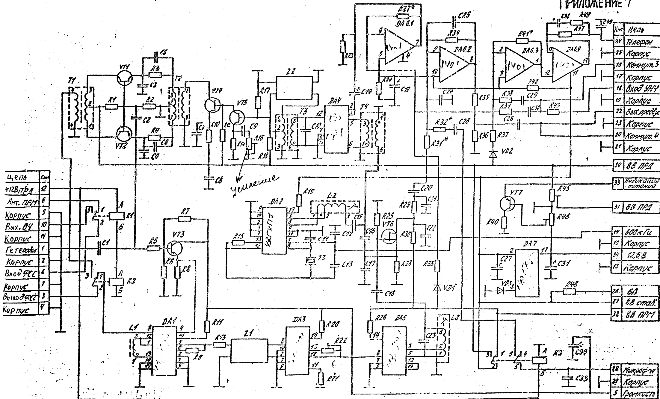
ИЗДАНИЕ „СЕВЕРОК-К“ УСТРОЙСТВО А2. СХЕМА ЭЛЕКТРИЧЕСКАЯ ПРИНЦИПИАЛЬНАЯ
