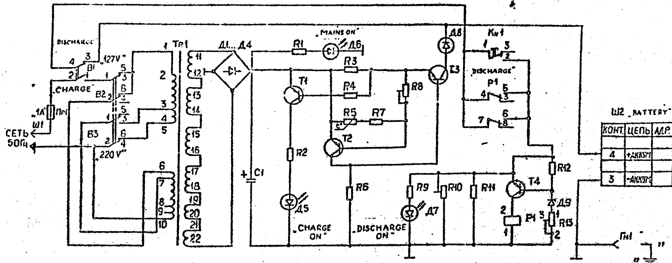
УСТРОЙСТВО ЗАРЯДНОЕ СЕТЕВОЕ. СХЕМА ЭЛЕКТРИЧЕСКАЯ ПРИНЦИПИАЛЬНАЯ
