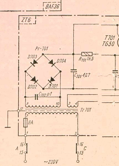
Schemat ideowy odbiornika radi
