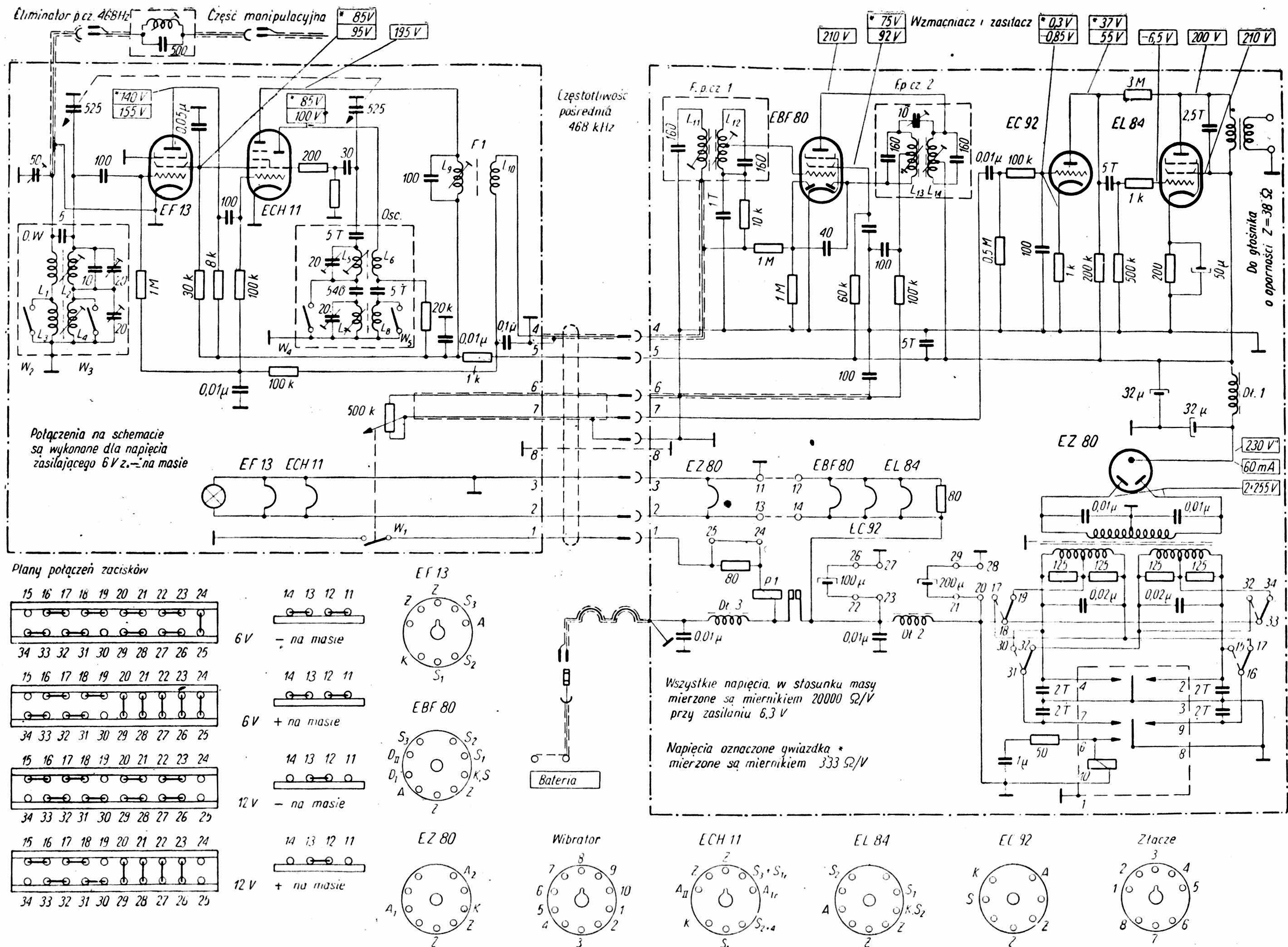
Rys. 4. Schemat ideowy odbiornika samochodowego „Rudelsburg“
