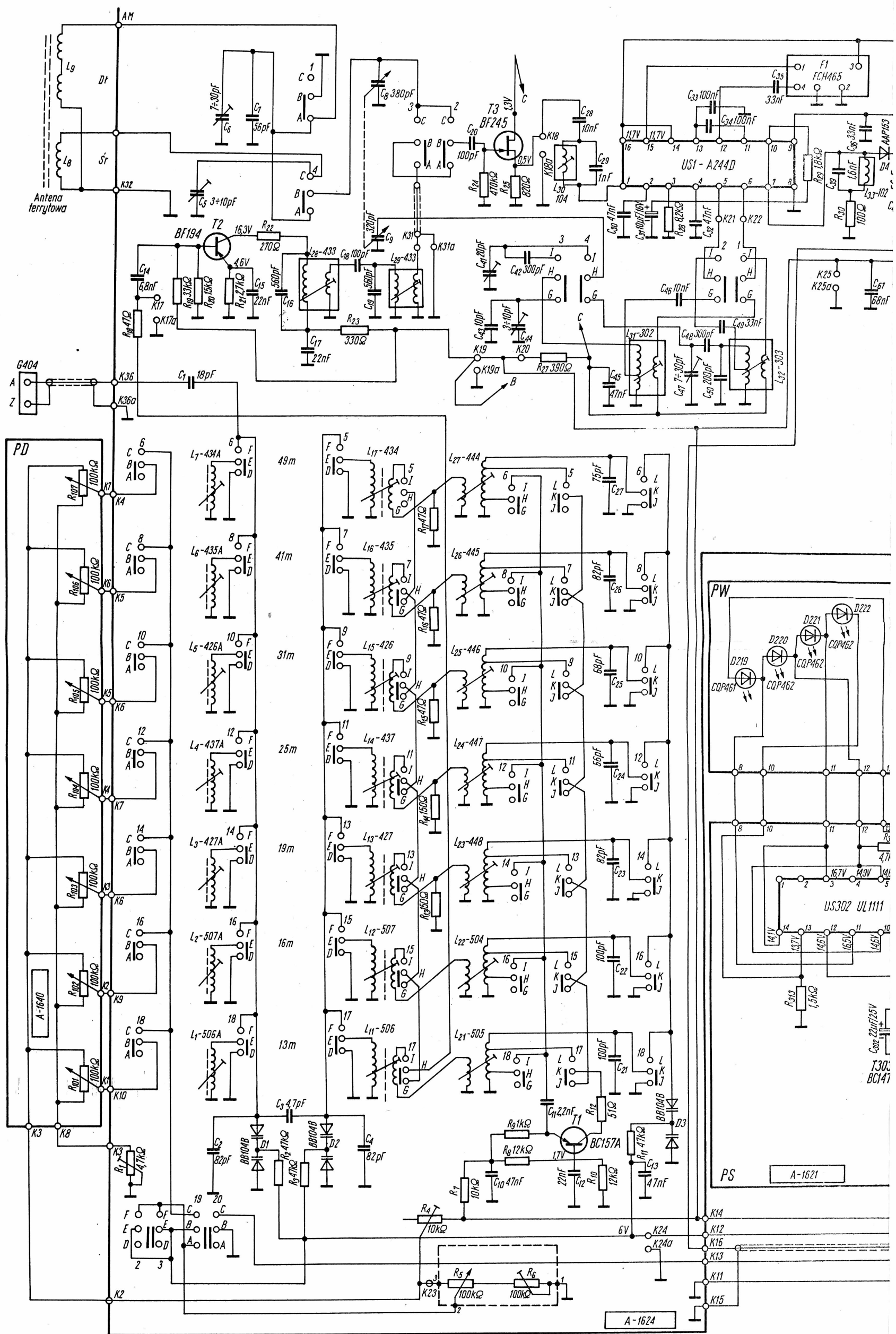
Rys. 28.42. Schemat ideowy tunera „Radmor” 5122 PD — blok dostrojenia, PS — blok sterujący wskaźnikami, PW — blok wskaźników
