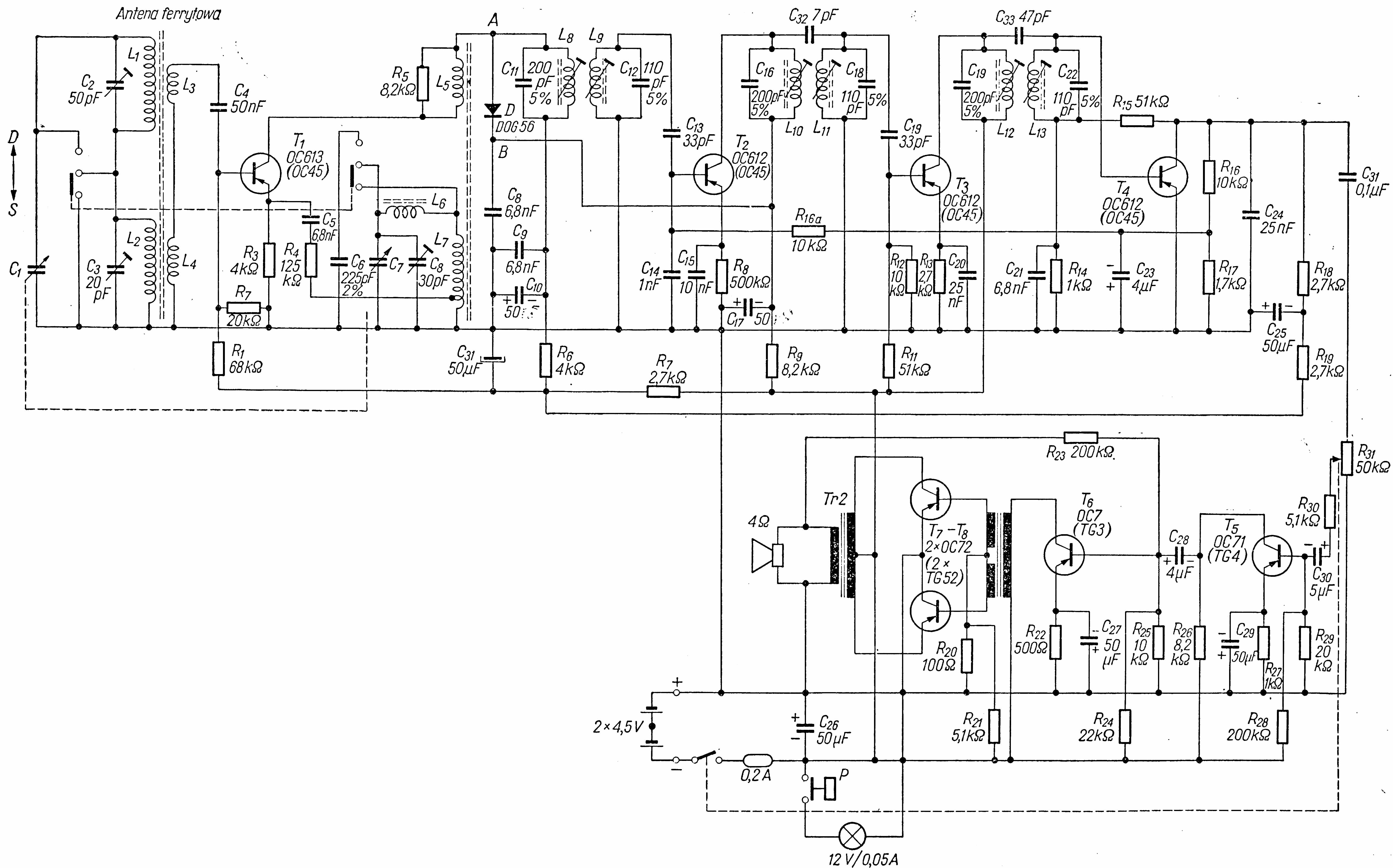
Schemat ideowy odbiornika „Szarotka TR” (kondensator C_{10} i C_{17} = 50 \mu F )
