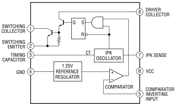
IC901 MC34063AM
