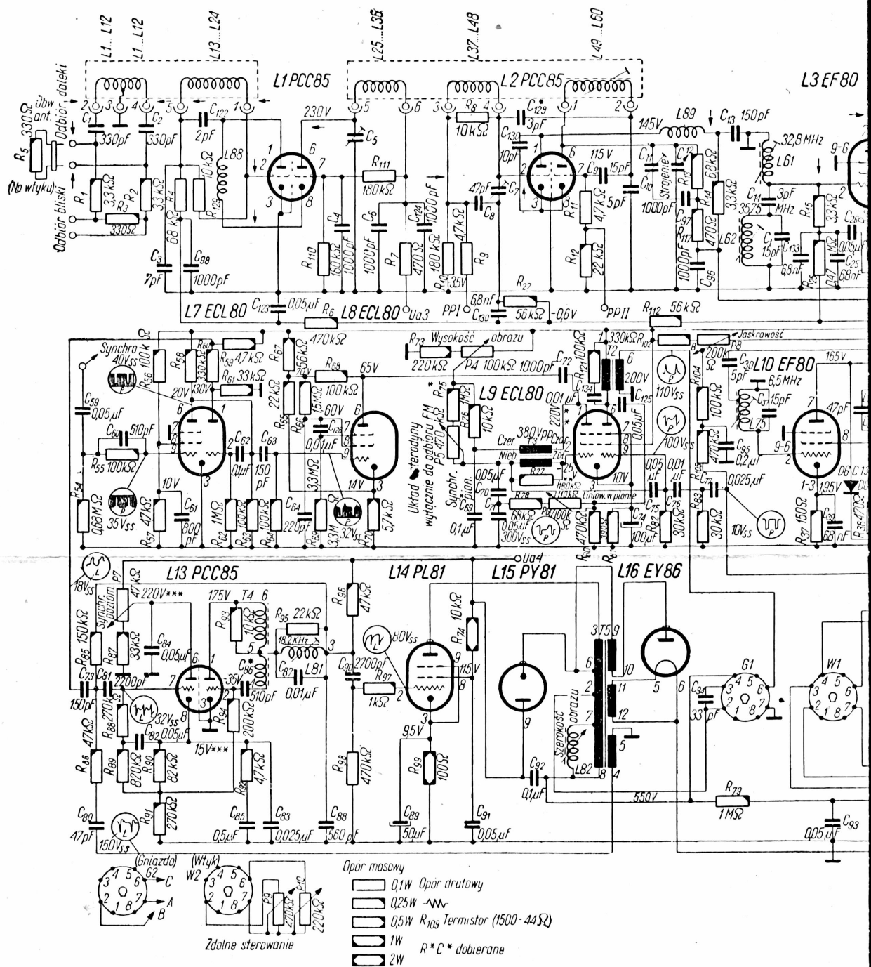
Rys. 70. Badanie wspólnej części toru wizji i fonii na przeno Strzałkami pokazano miejsca dołączenia
