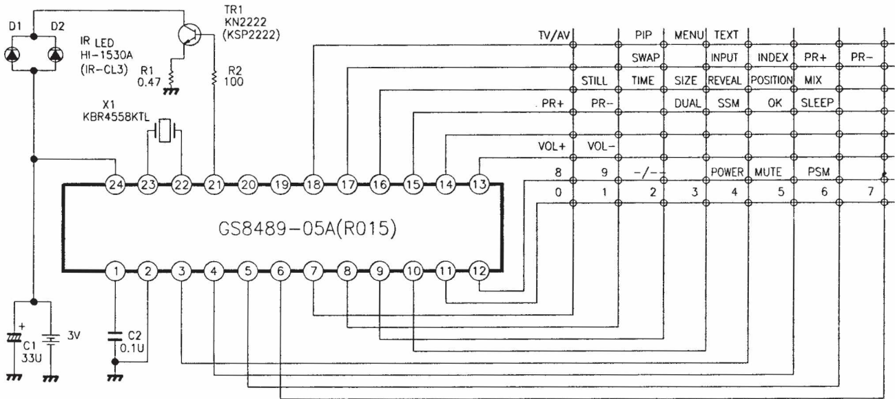
Принципиальная схема пульт ДУ
