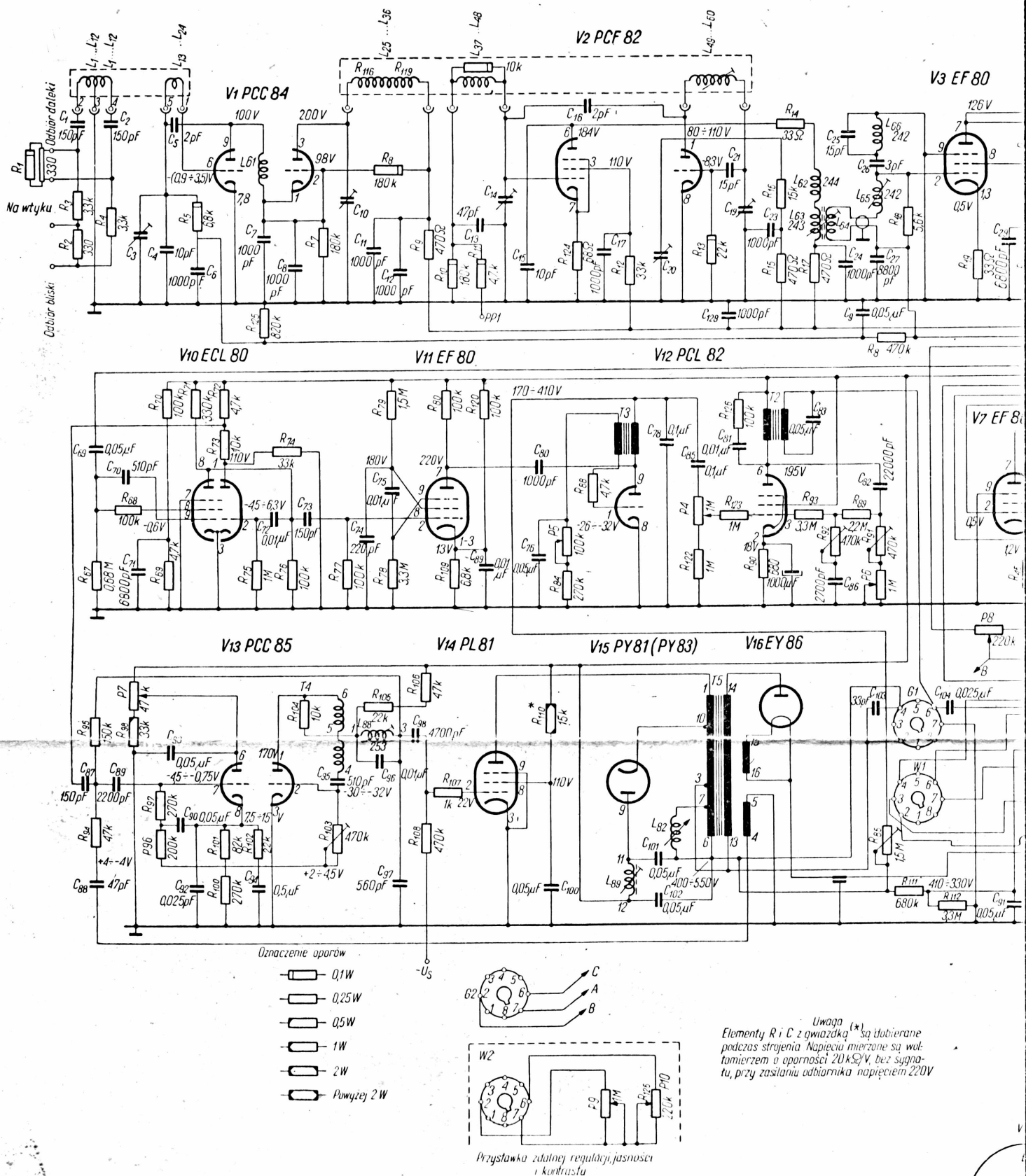
Rys. 6. Schemat ideowy odbiornika „Neptun”.
