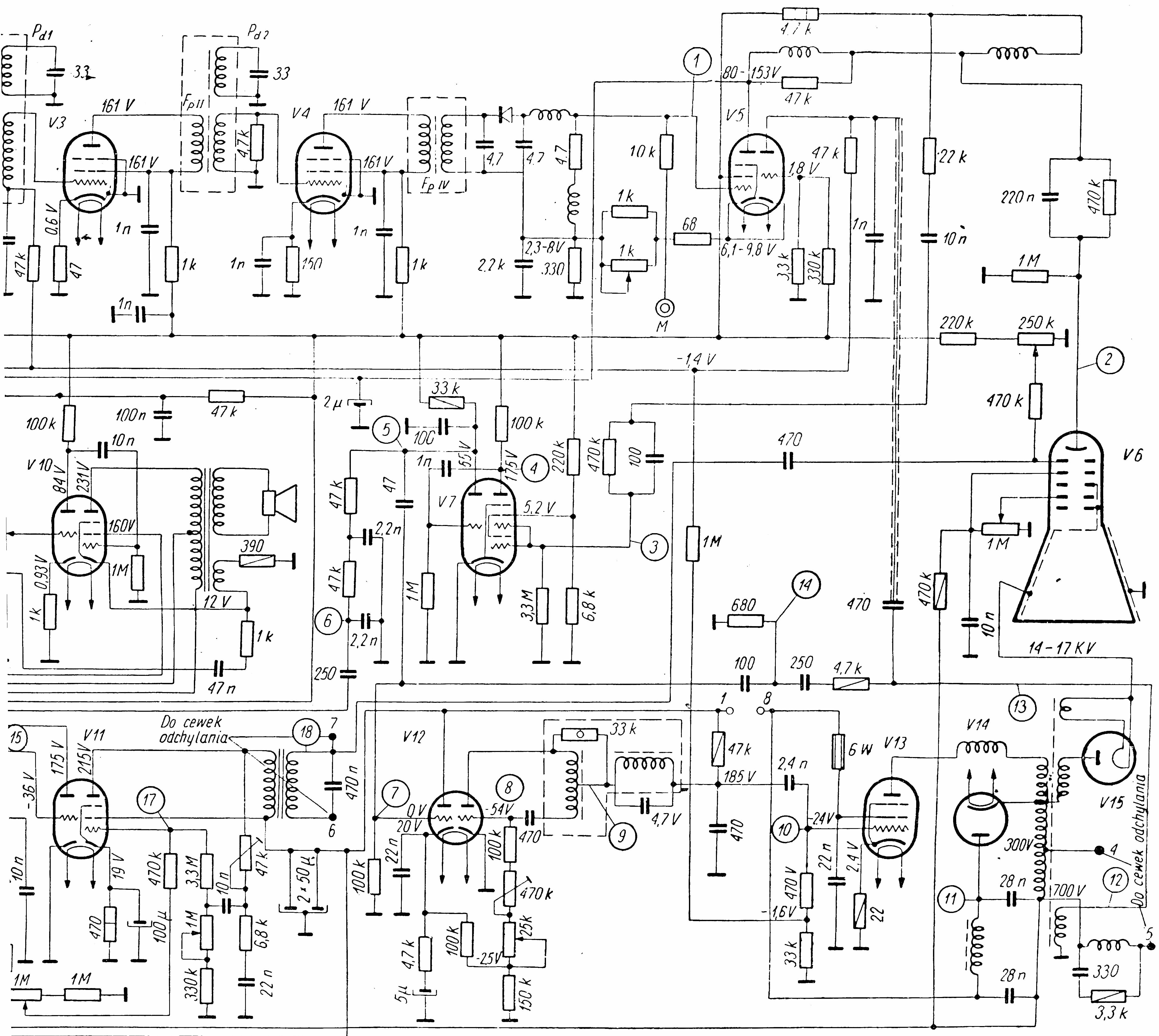
Schemat ideowy telewizora Orion „AT 504”
