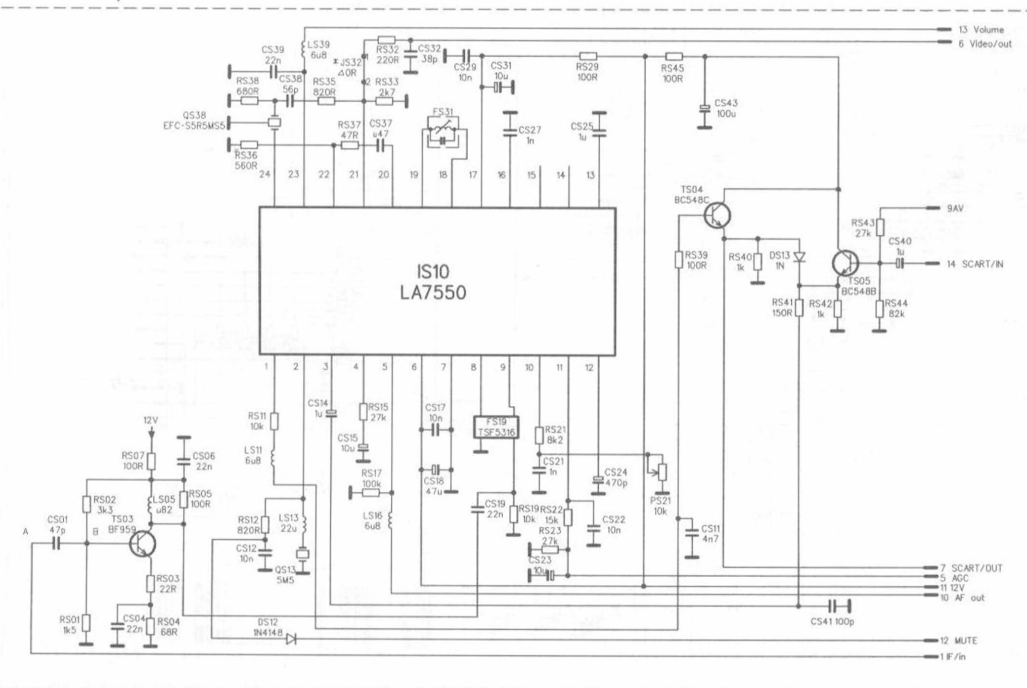
IF Amplifier 2600
