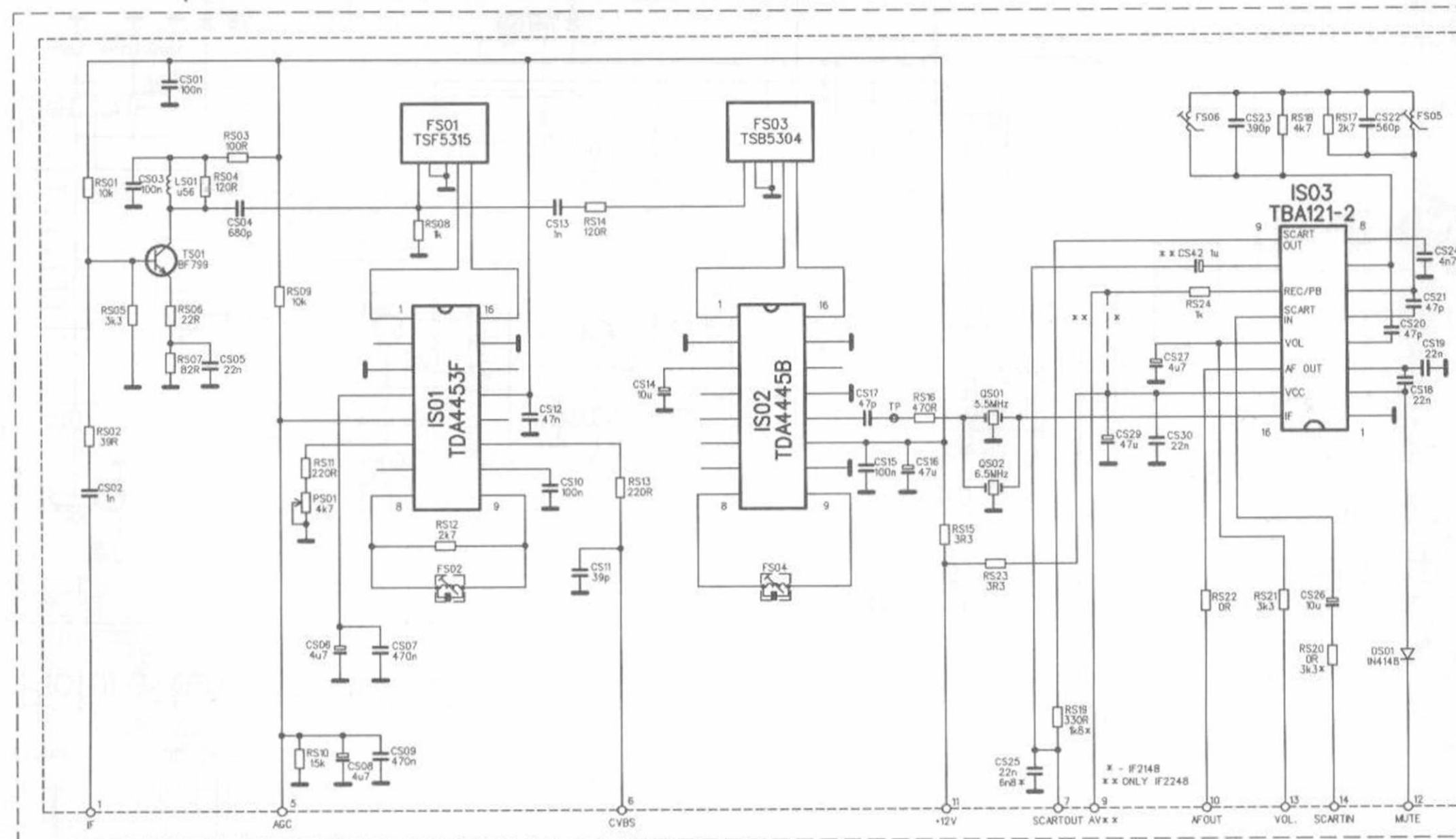
IF Amplifier 2148, 2248
