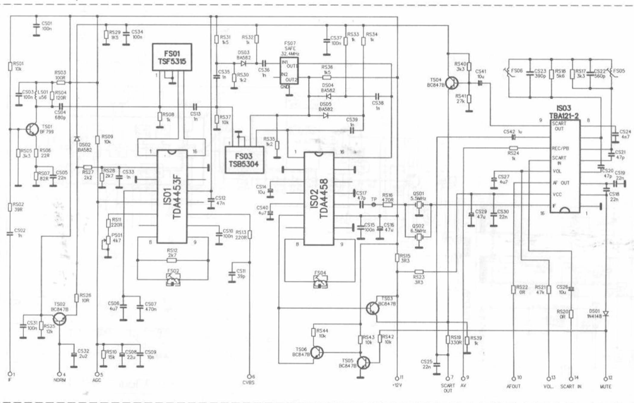
IF Amplifier 2149
