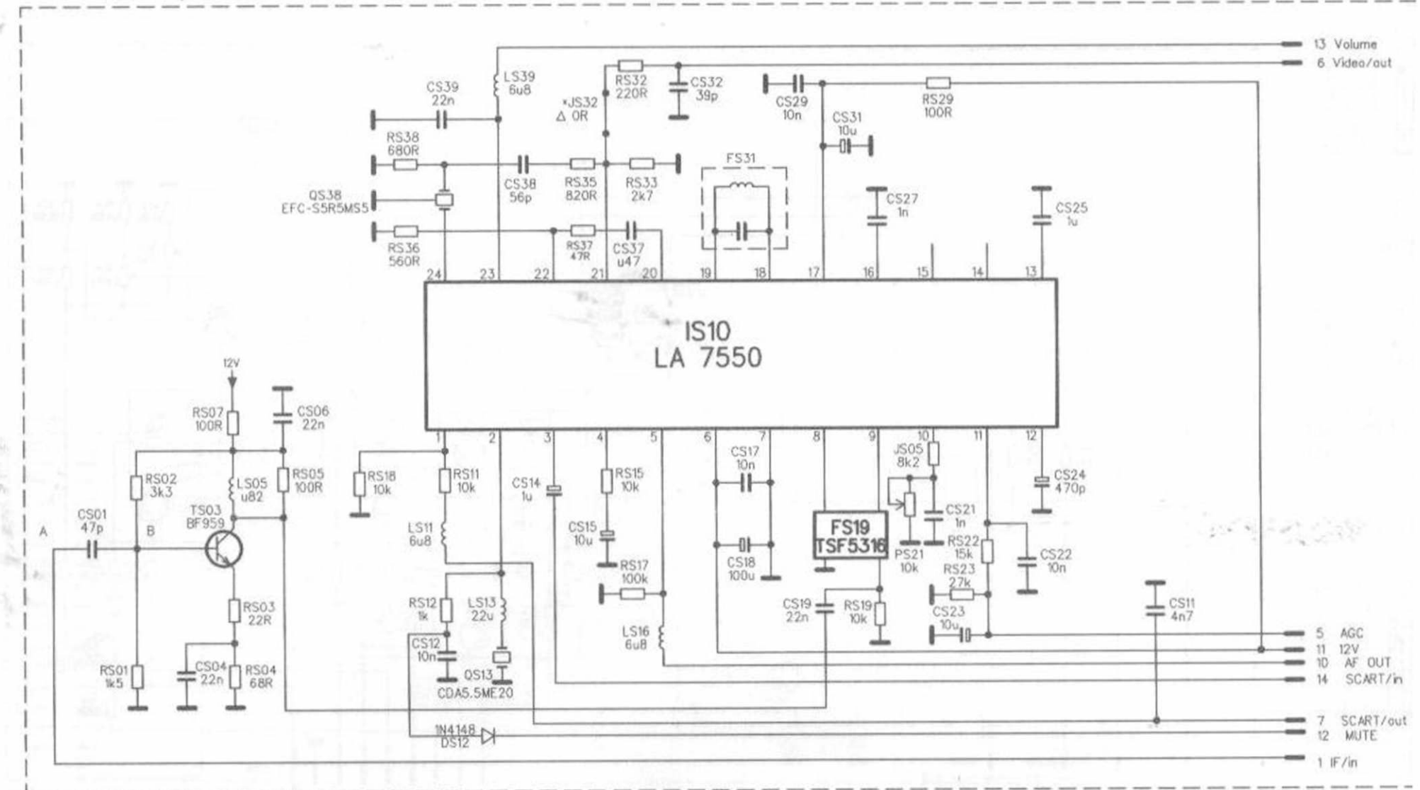
IF Amplifier 2109
