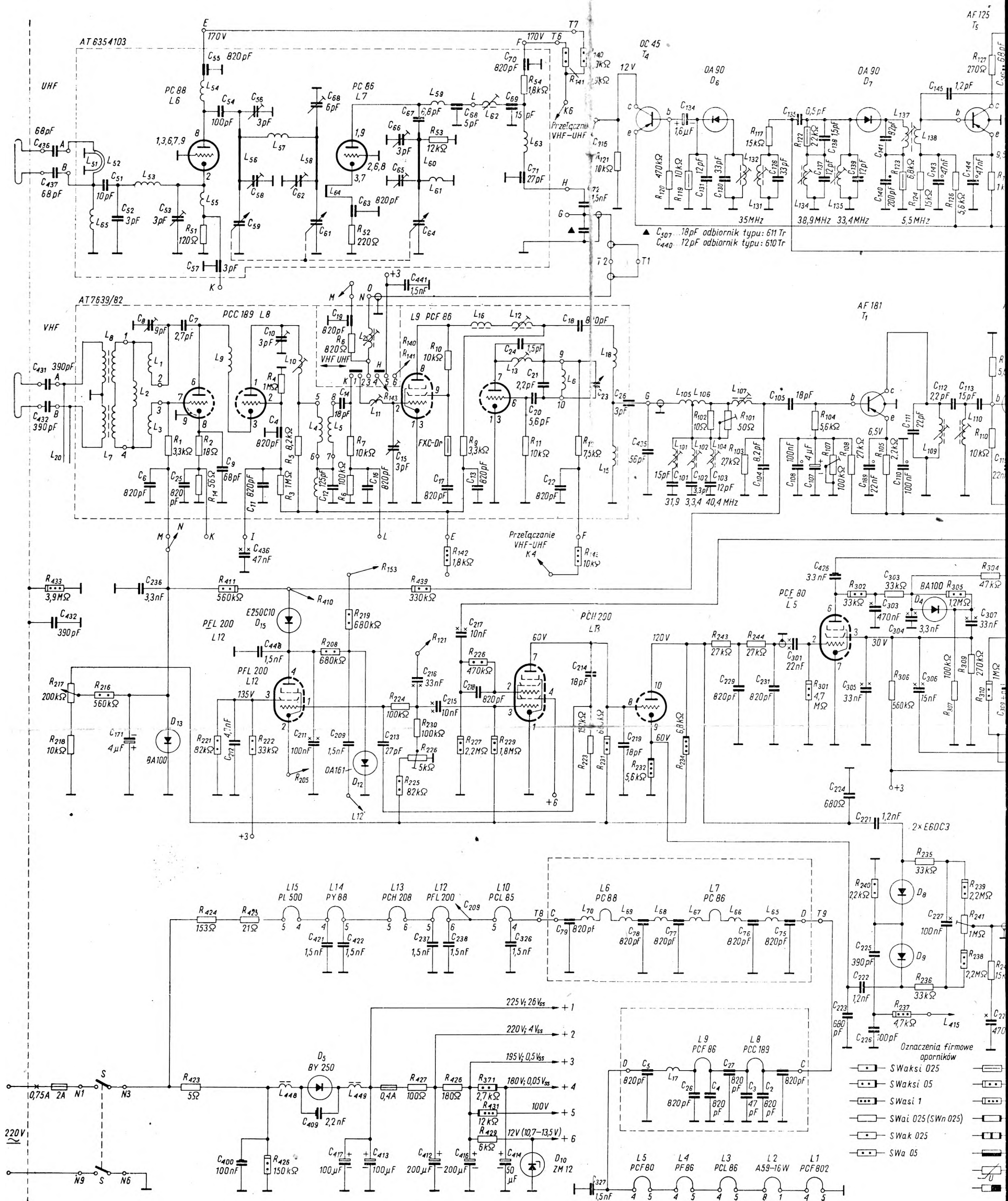
Rys. XVII.95. Schemat elektryczny odbiornika lampowo-tranzystorowego
